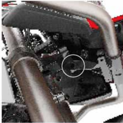
Ajuste de la altura del haz del faro
