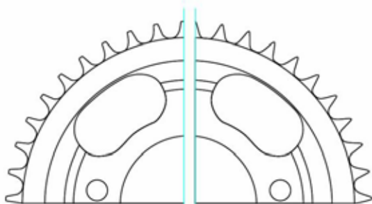
Dientes corona correctos
